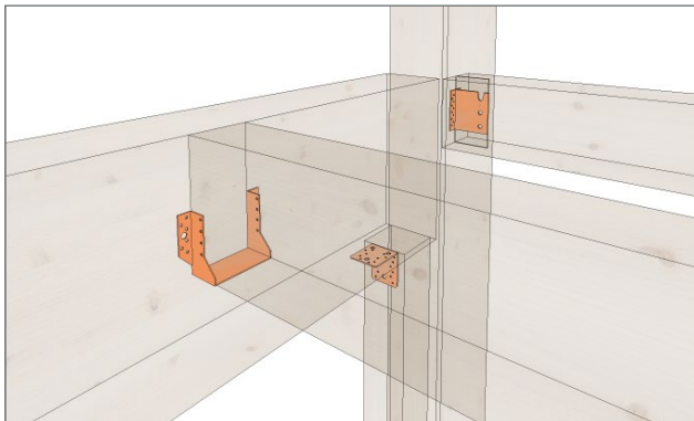
Bild 30. Balkenanschlüsse
