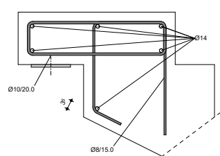
Schnitt Ausklinkung
