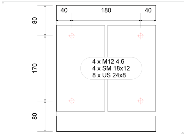
Bild 26. Bemaßung Schraubenbild
