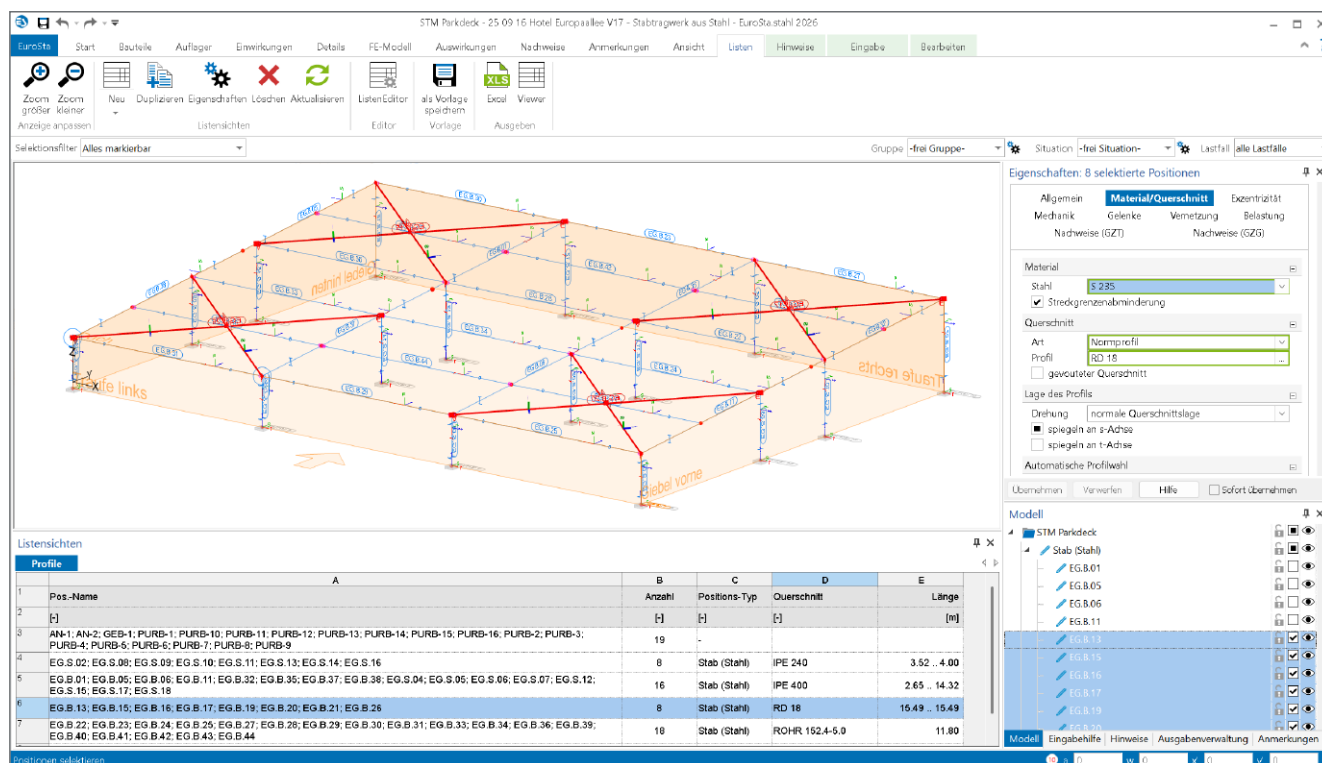
Bild 1. 3D-Stabwerksmodell in EuroSta.stahl mit Listensicht zur Auswertung der Querschnittsprofile
