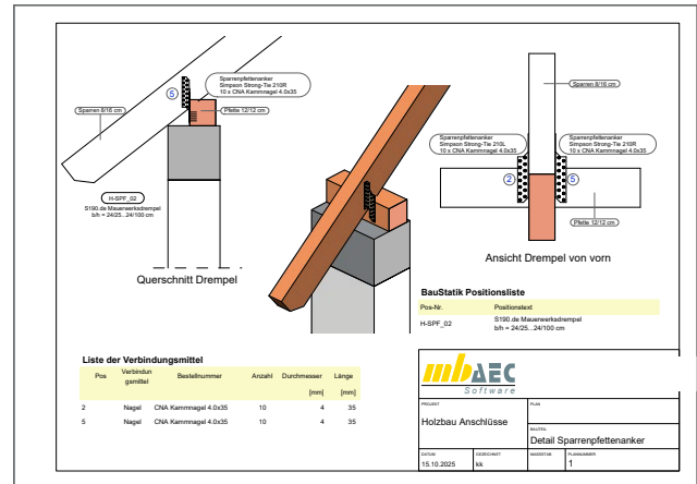
Bild 38. Detailplan Sparrenpfettenanker
