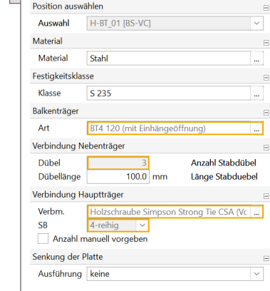
Bild 33. Balkenträger (Einhängeöffnung)
