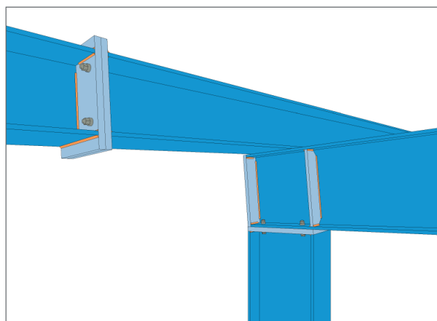
Bild 22. Schrauben und Schweißnähte
