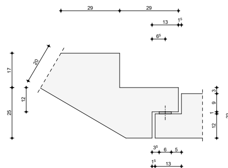
Bild 1. Systemskizze eines Treppenanschlusses
