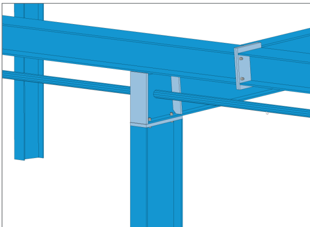
Bild 2. Rahmenecke und Stirnplattenstoß
