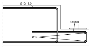
Schnitt Konsole
