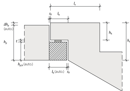
Bild 3. Grafische Hilfe zur Option "UK Treppe und UK Podest auf gleicher Höhe"
