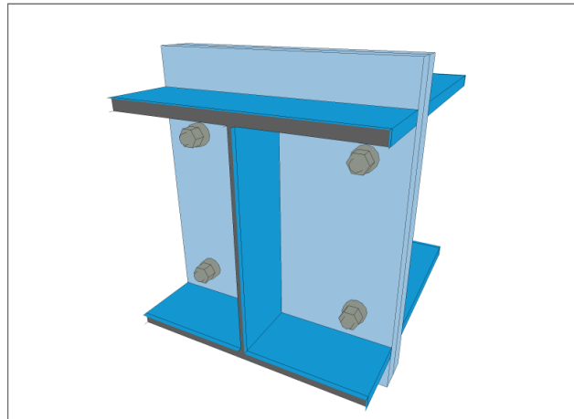
Bild 24. Schraubenbild
