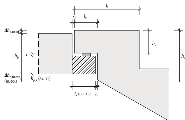
Bild 4. Grafische Hilfe zur Option "Versatz"
