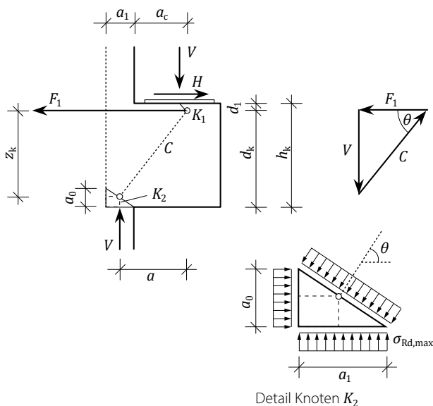
Bild 9. Fachwerkmodell nach Reineck
