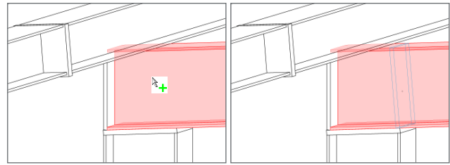
Bild 14. Erzeugung Rippen
