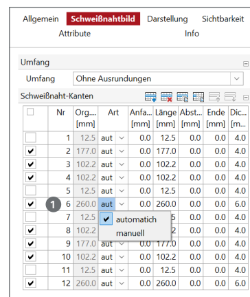
Bild 29. Eigenschaften Schweißnahtbild
