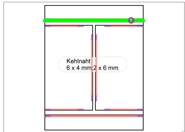
Bild 28. Bearbeitung Schweißnahtbild
