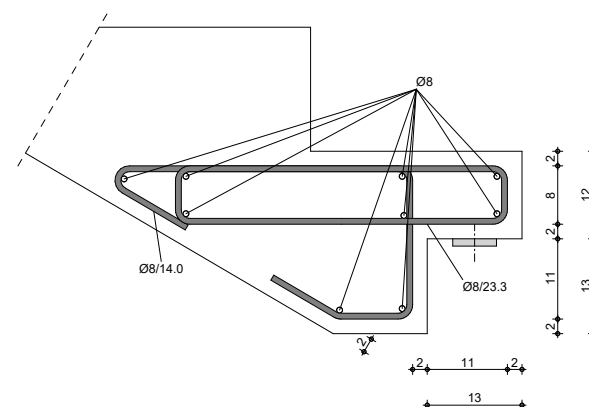
Bild 8. Ausgabebeispiel einer Bewehrungsskizze
