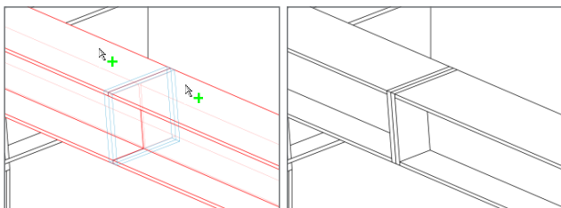
Bild 12. Erzeugung Stirnplattenstoß markieren der Bauteile
