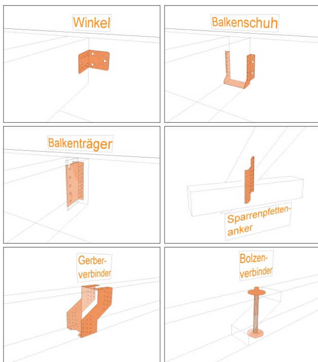
Bild 31. Übersicht Holzbauelemente
