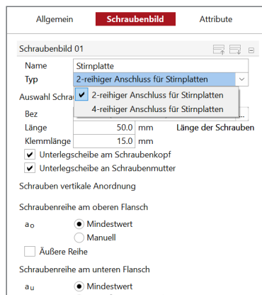
Bild 25. Eigenschaften Schraubenbild
