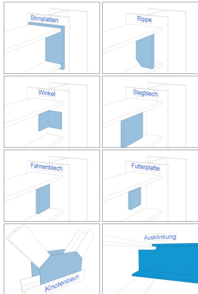
Bild 3. Übersicht „Stahlbau-Anschlüsse“
