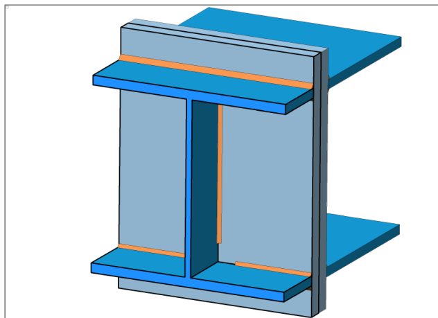
Bild 27. Schweißnahtbild
