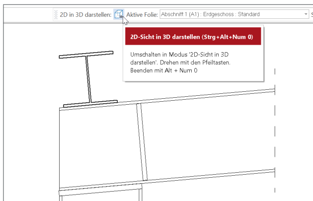
Bild 18. 3D-Darstellung aktivieren
