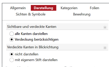
Bild 19. Sichtdarstellung einstellen
