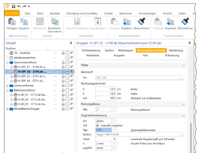
Bild 34. BauStatik Eingabe
