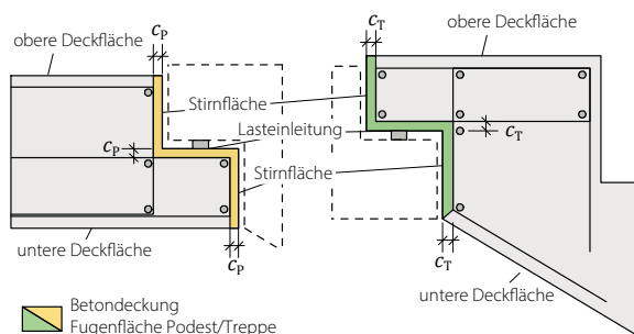
Bild 5. Grafische Hilfe zur „Fugenfläche“
