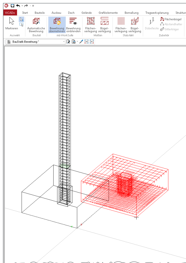
Bild 1. Bewehrungsübernahme in ViCADO
