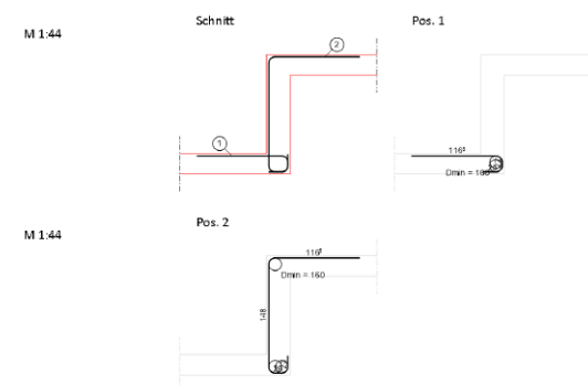
Bild 13. Nachweis für Deckenversatz aus MicroFe mit S292.de
