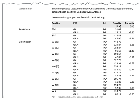
Bild 5. Lastübergabe-Protokoll: Lastsummen
