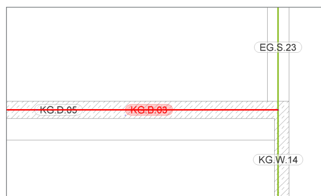
Bild 4. Idealisiertes Strukturmodell
